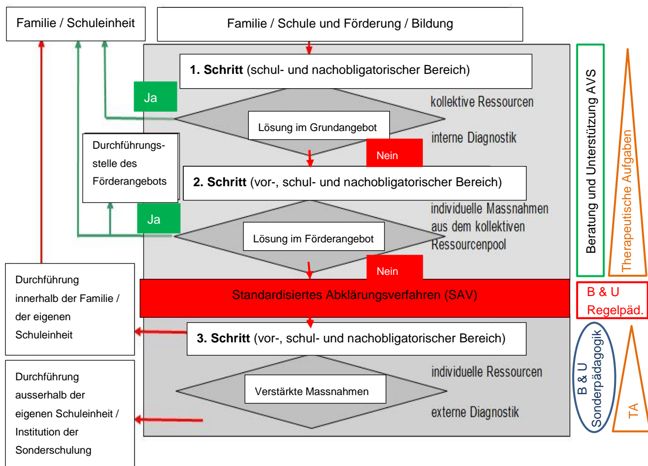
Abbildung 2: Das Kaskadenmodell
